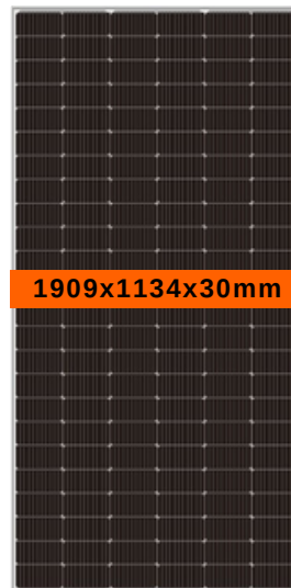
MÓDULO FOTOVOLTAICO MONO 460WP 120 CÉLULAS CLASE A
